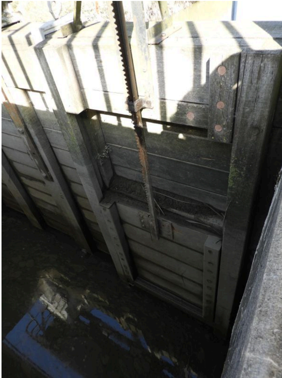
La vantelle aménagée dans la vanne verticale.
