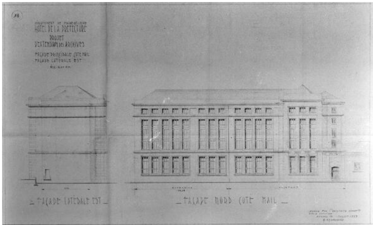
Département de Maine-et-Loire. Hôtel de la Préfecture. Extension des Archives départementales. 3e tranche : façade principale côté mail, façade latérale est, plan, par H. Enguehard, 1959, éch. 1 : 100. (Archives départementales de Maine-et-Loire ; 233 W 158).
