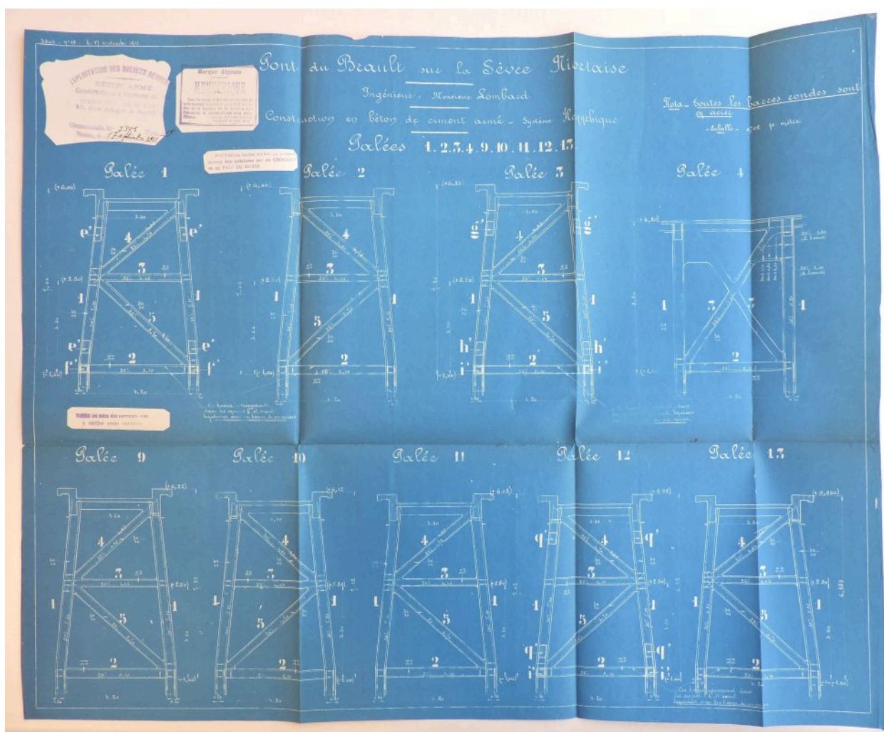
Dessin d'exécution des travaux de construction du pont, élévations des palées, 1912.
