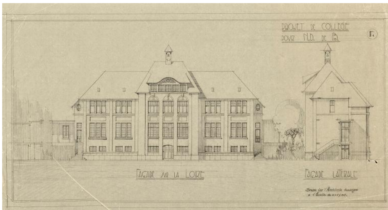
Projet de collège pour Notre-Dame de Béhuard. Façade sur la Loire et façade latérale. n.s. n.d.
