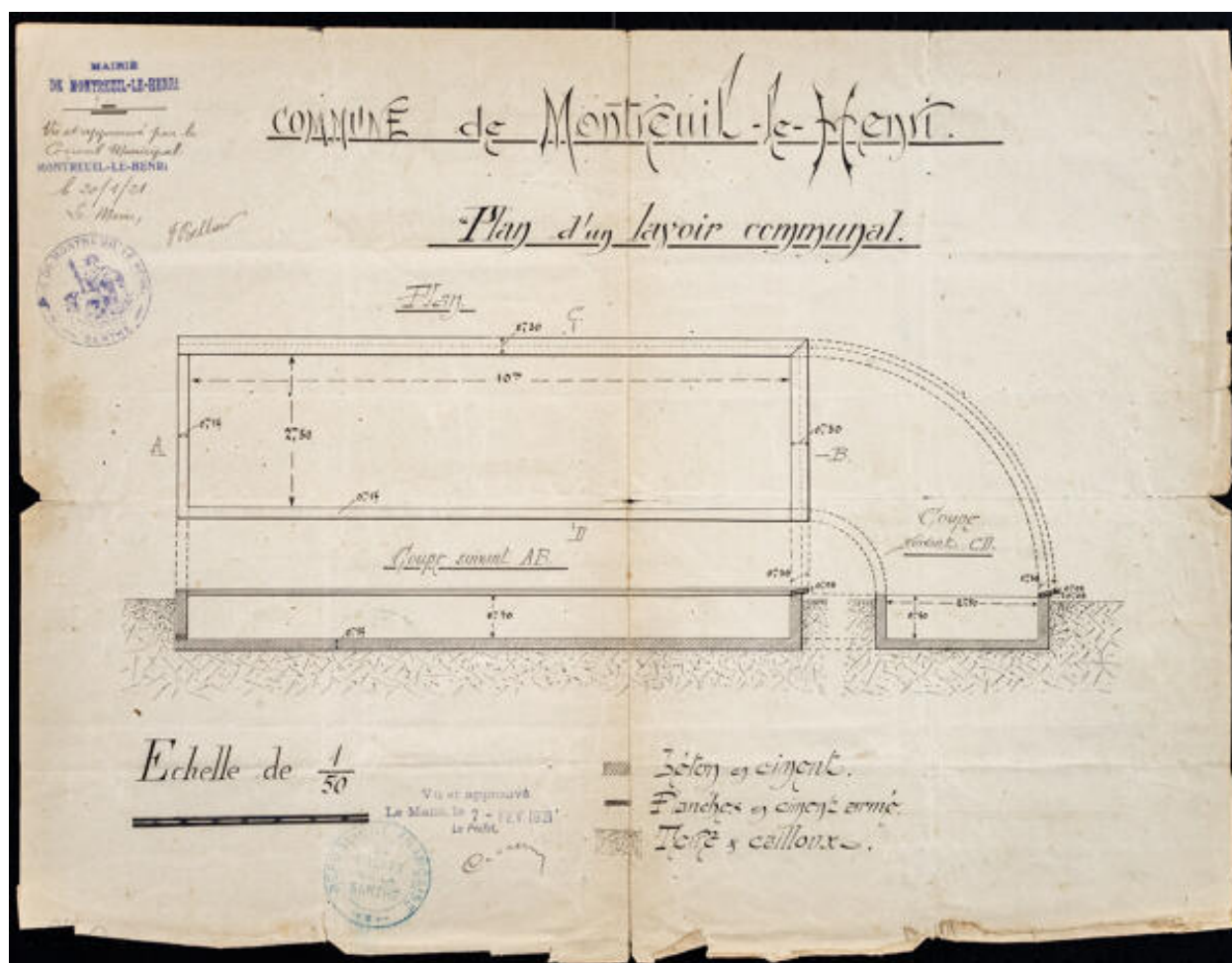
Lavoir communal de Montreuil-le-Henri : plan au sol et coupes, 1921.
