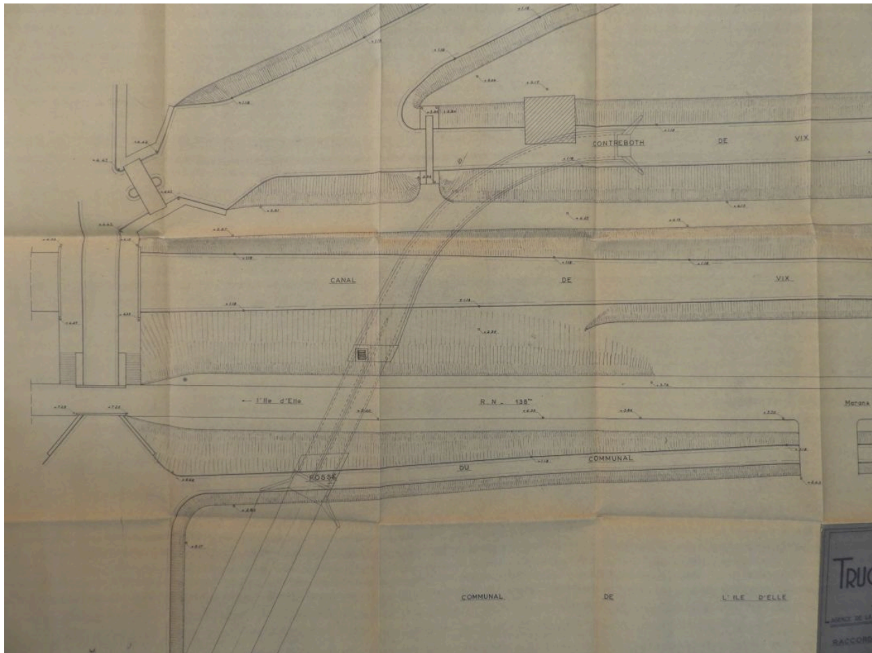
Plan du projet de siphon reliant la Vendée au Contrebot, par l'entreprise Trucheret-Tansini, 18 août 1959.
