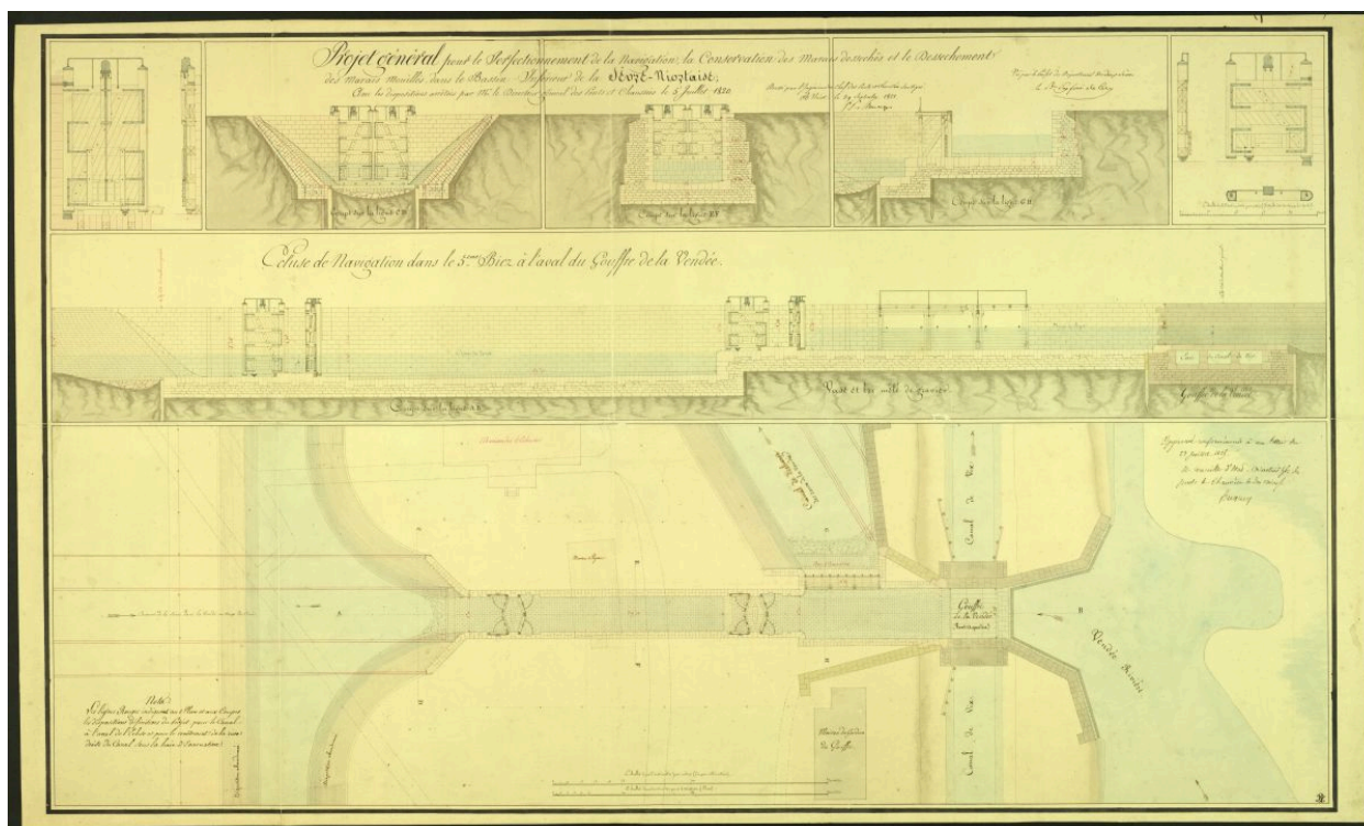
Projet d'écluse de navigation au Gouffre, par Mesnager, 1821.
