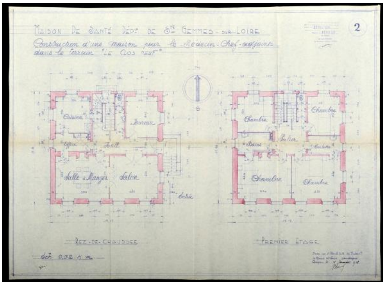
Construction d'une maison pour le Médecin-Chef-adjoint dans le terrain ""Le clos neuf"". Rez-de-chaussée et premier étage, par Ernest Bricard. 1928. (Archives départementales de Maine-et-Loire, 4 N).
