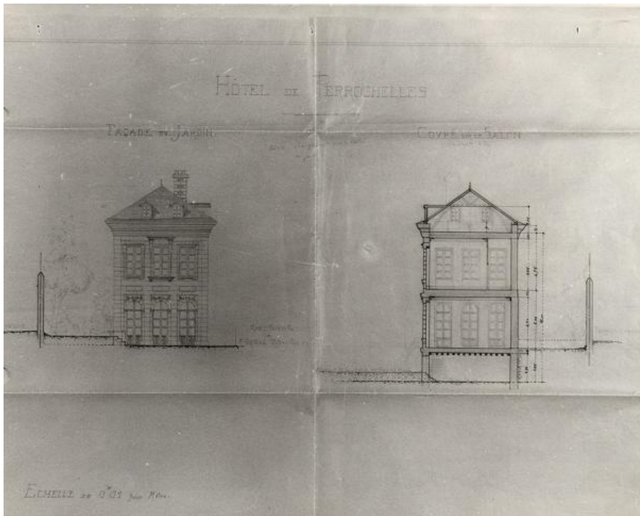
Elévation latérale et coupe transversale gauche, projet, par l'architecte Auguste Martin, fin 19e siècle, éch. 1 : 100. (Collection particulière, M. Pousset).
