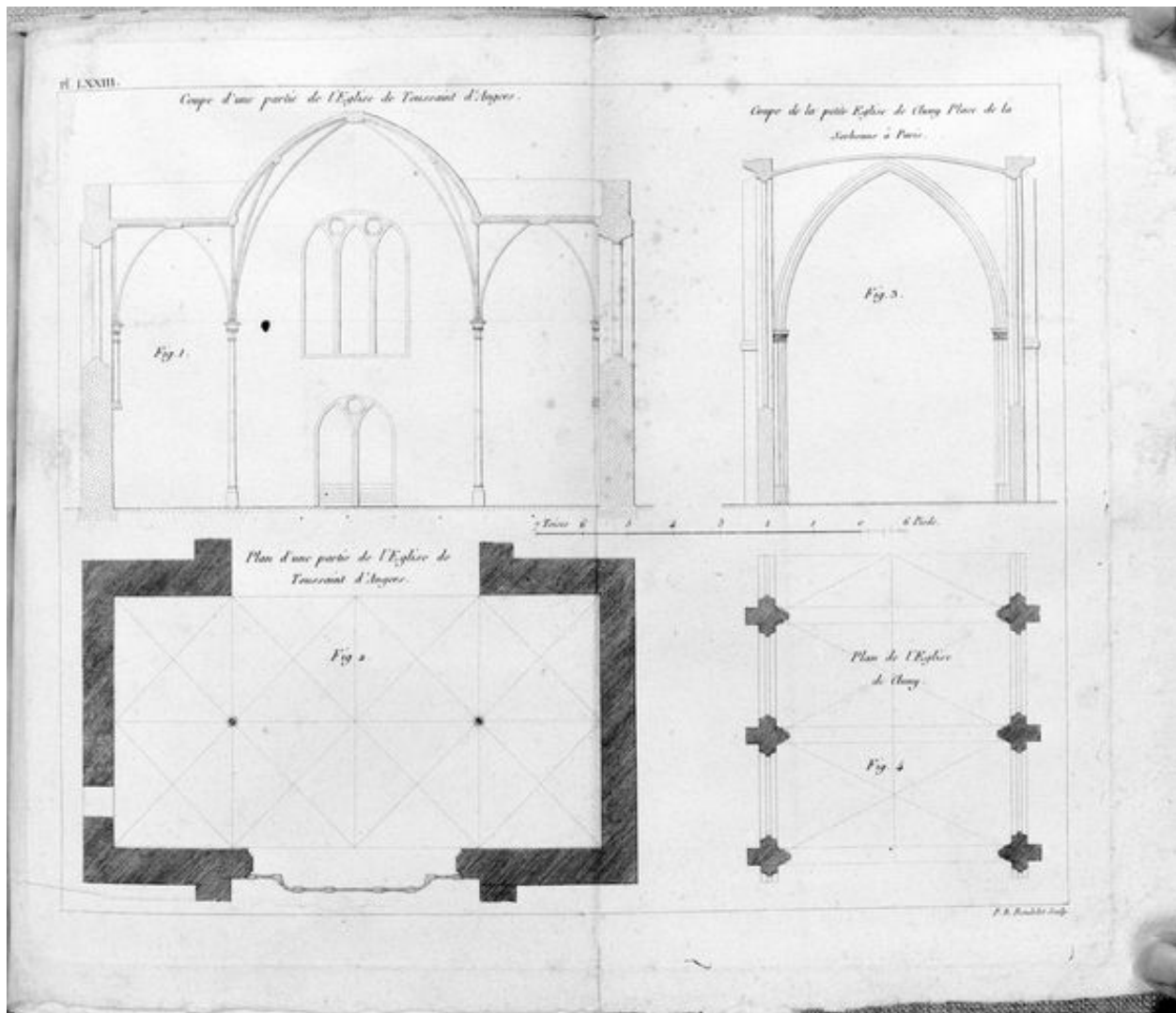
Abbatiale, plan et coupe du transept, [v. 1821]. Dessin, in : BODIN, J.-F. "Recherches historiques sur l'Anjou et ses monuments. Angers et le Bas-Anjou", Saumur, Degouy, 1821-1823, t. 1.
