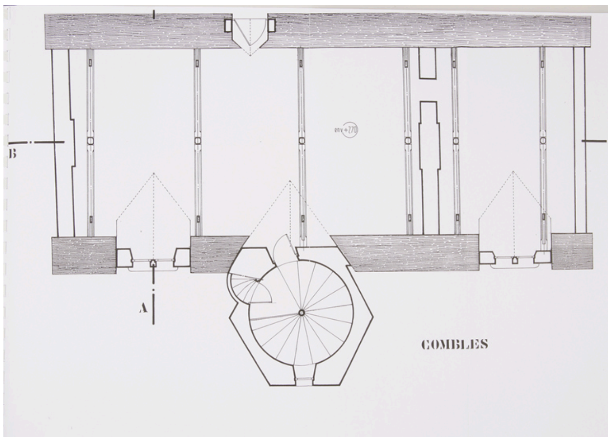
Plan du comble.
