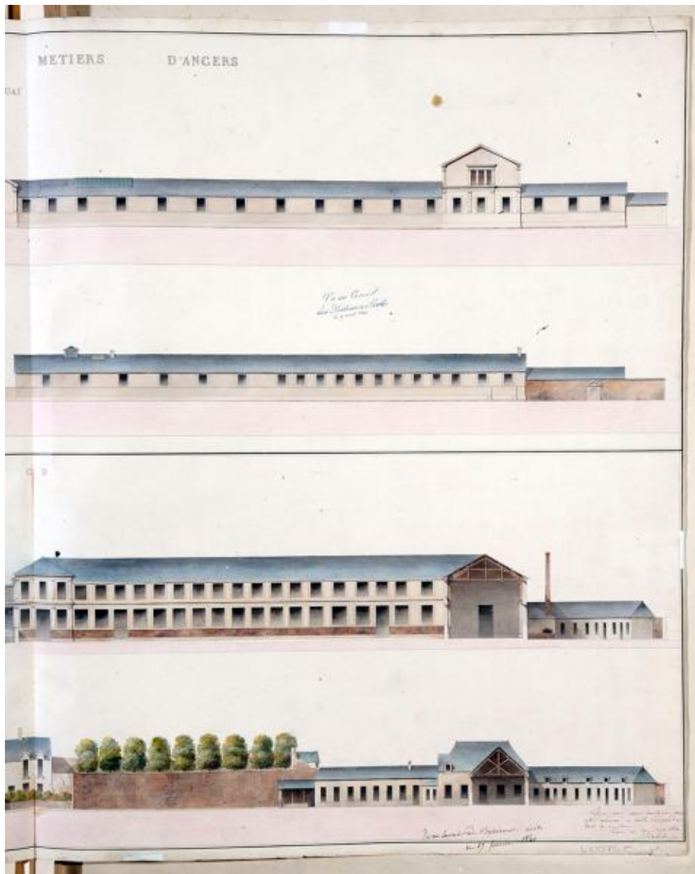
Ecole royale des Arts-et-Métiers. Façade sur le quai. Coupe sur la ligne CD [sud-nord le long de l'aile Est du cloître et du bâtiment d'ajustage]. Etat projeté. Etat actuel, 1839. Détail : partie droite de la planche.
