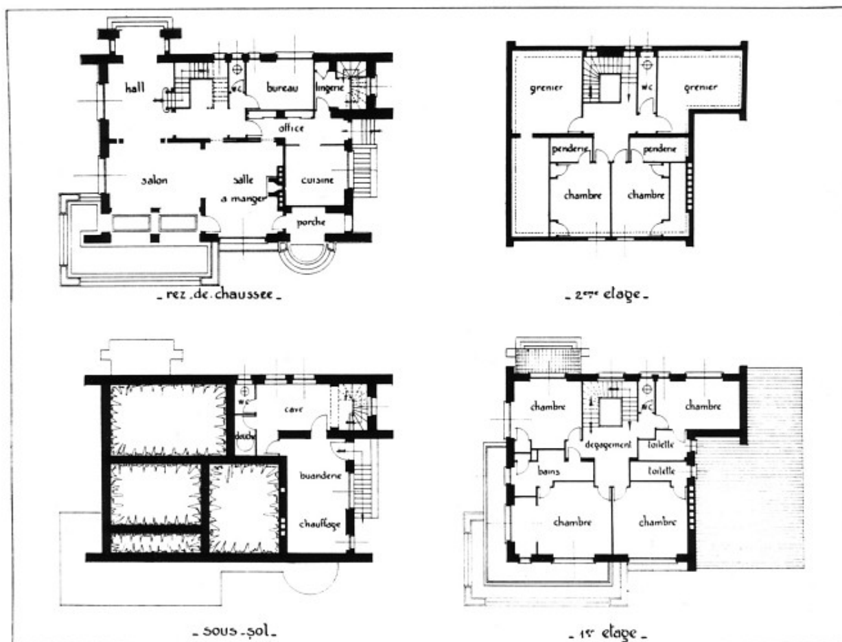
Plans des rez-de-chaussée, sous-sol, 1er et 2e étages de la villa Blanche.
