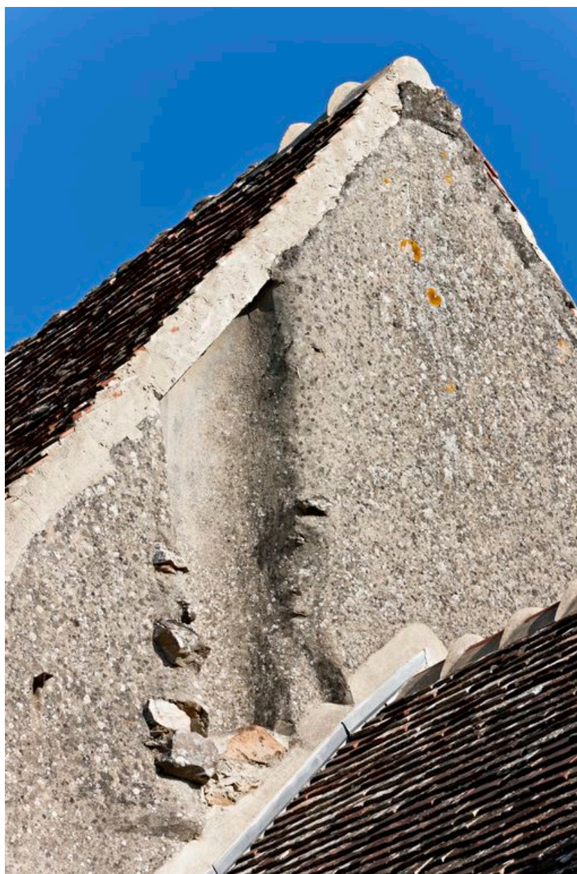
Détail du vestige d'un conduit de cheminée cylindrique.
