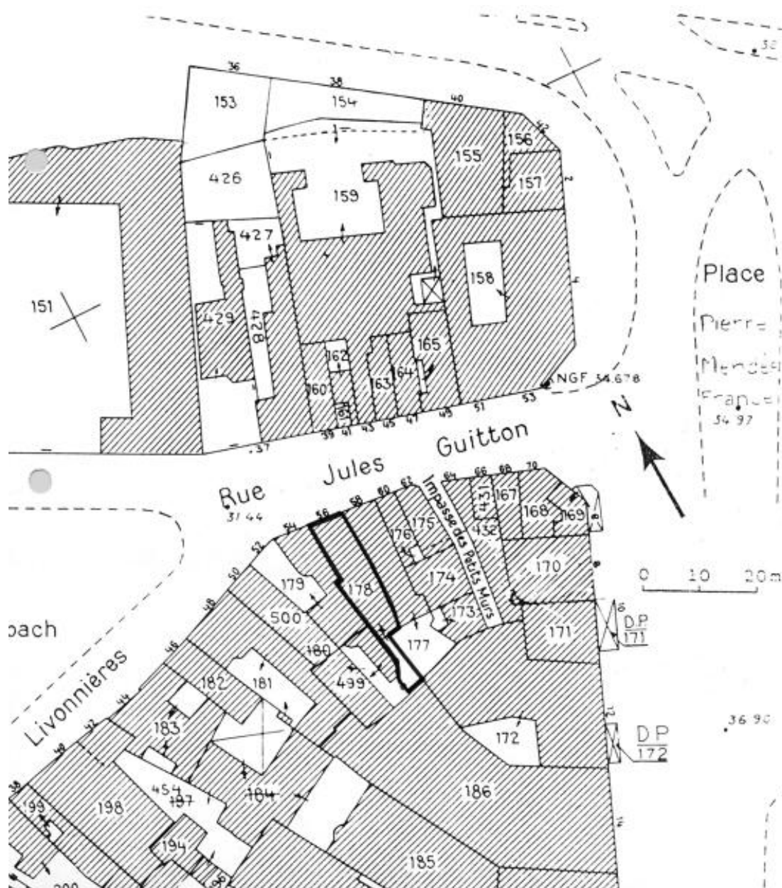
Plan-masse et de situation. D'après le plan cadastral, 1980, section BR, parcelle 178, éch. 1 : 1 000, agrandi.
