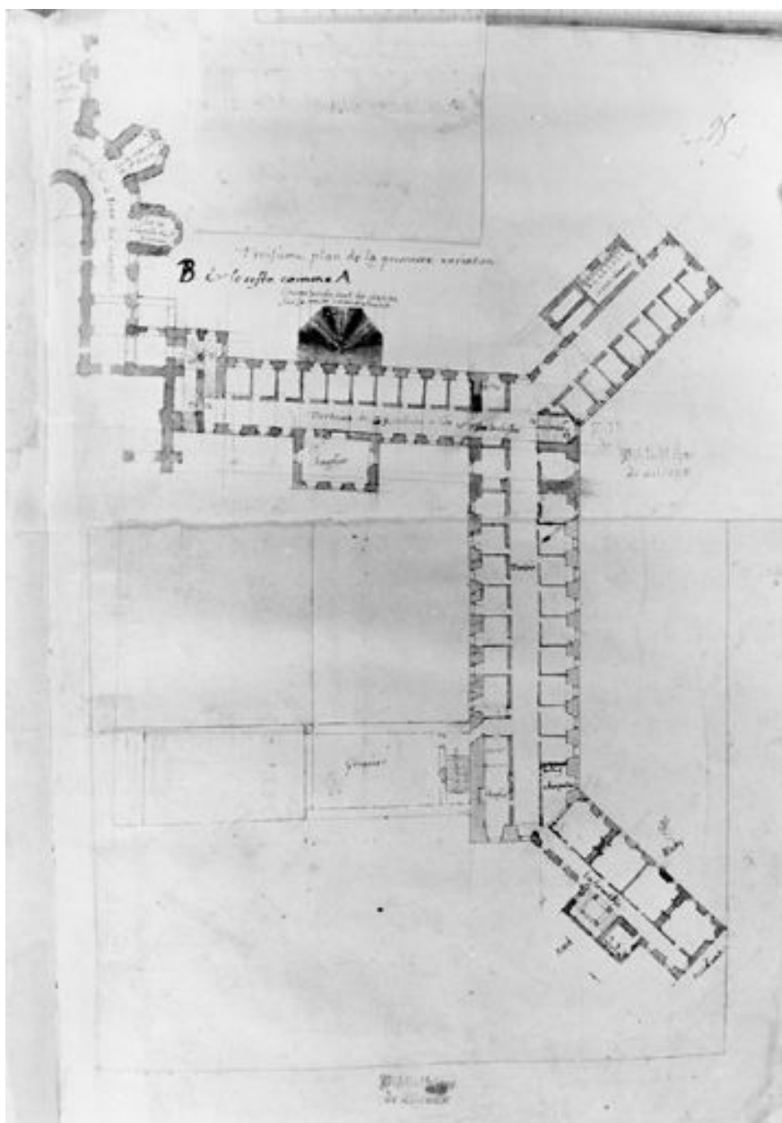
Projet "B" : plan d'ensemble avec la salle du chapitre formant avant-corps, étage carré au-dessus du réfectoire, 1685. (Bibliothèque municipale de Meaux ; Ms. 44, f. 95).
