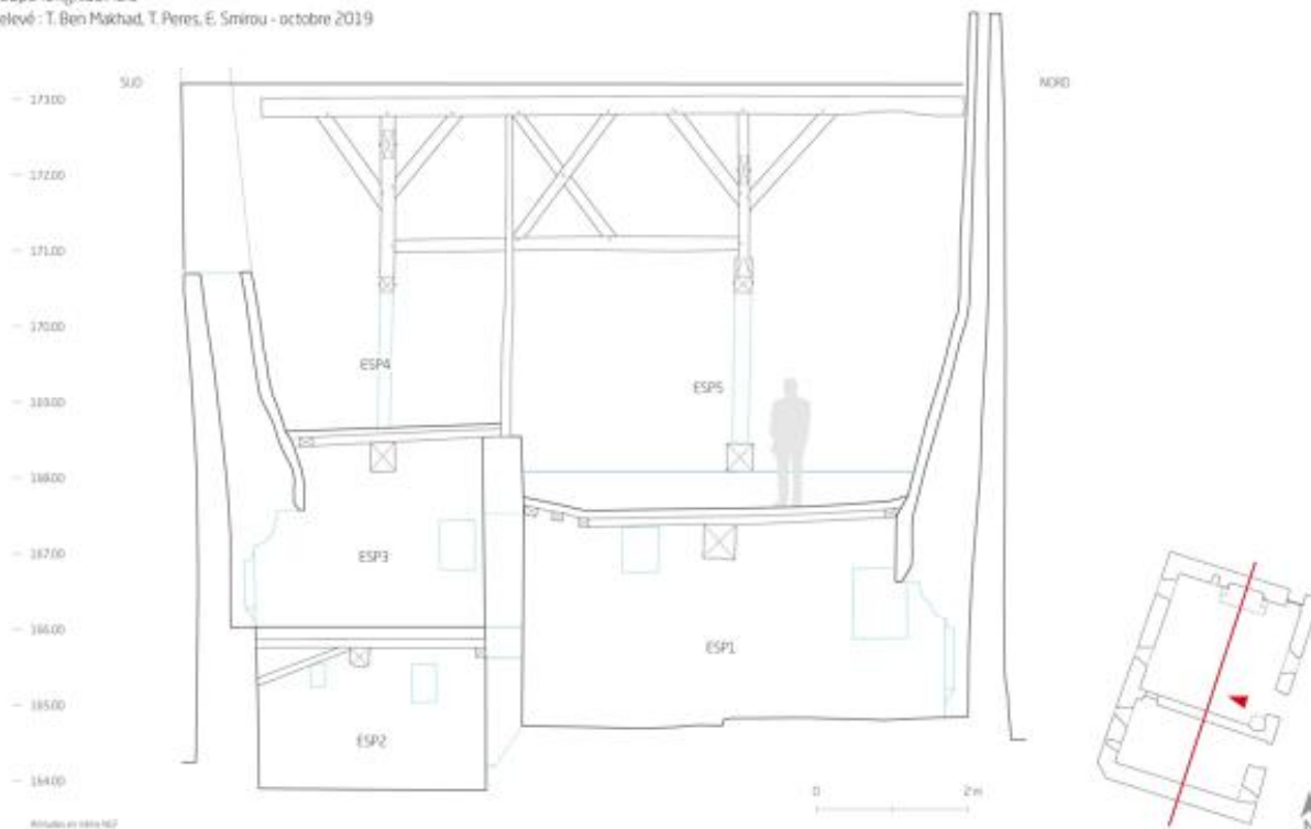
Coupe longitudinale de la maison de Bignon.
