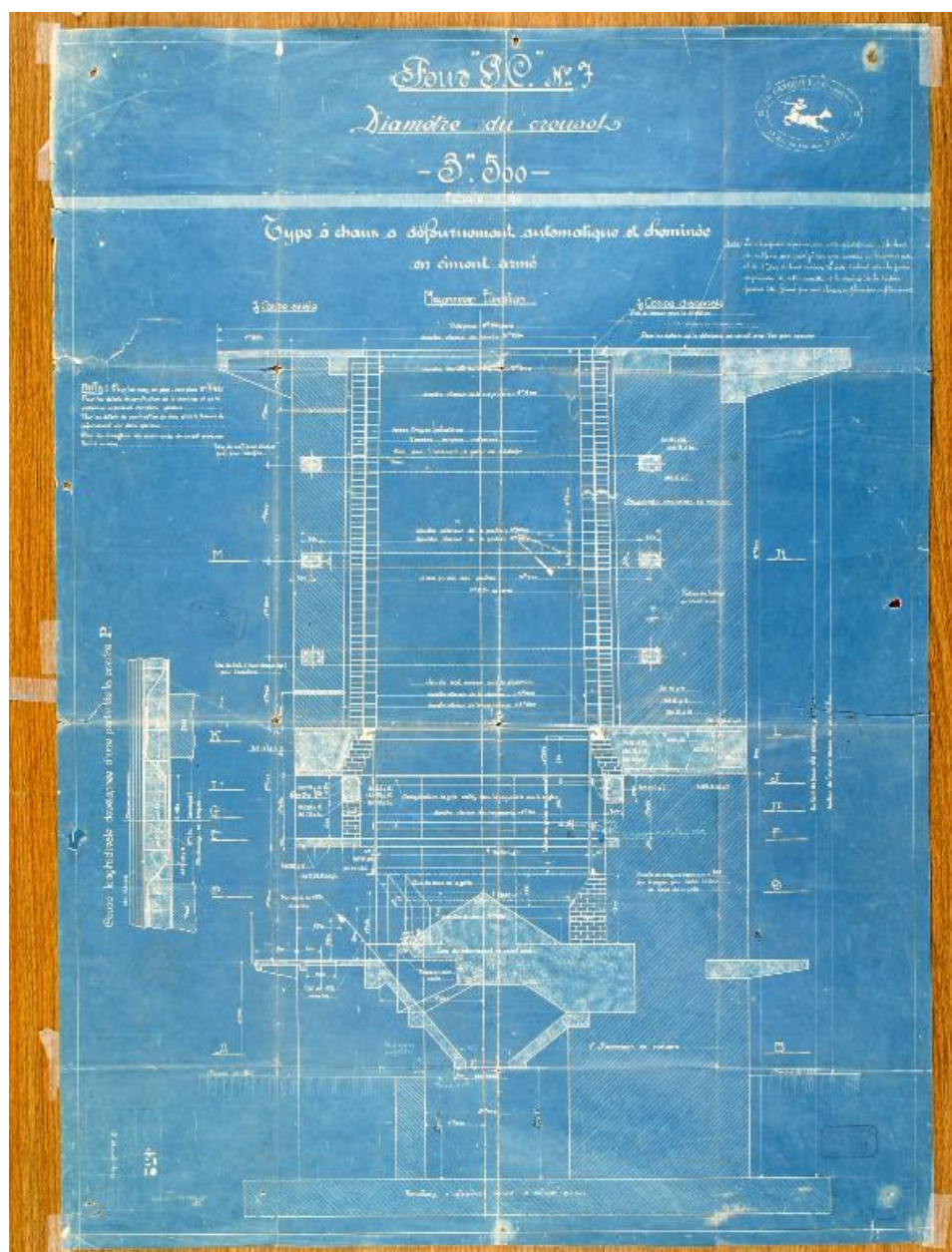
Four P.C. n°7, type à chaux à défournement automatique et cheminée, plan, par Charles Candlot, Ingénieurs constructeurs, 1919
