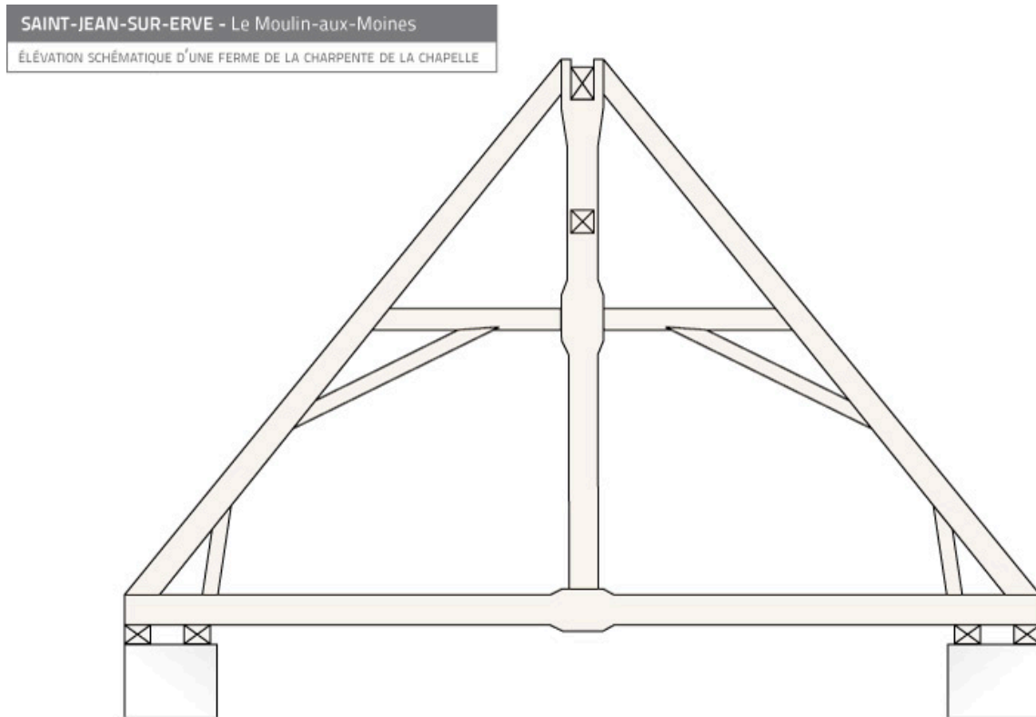
Élévation schématique d'une ferme de la charpente de la chapelle.
