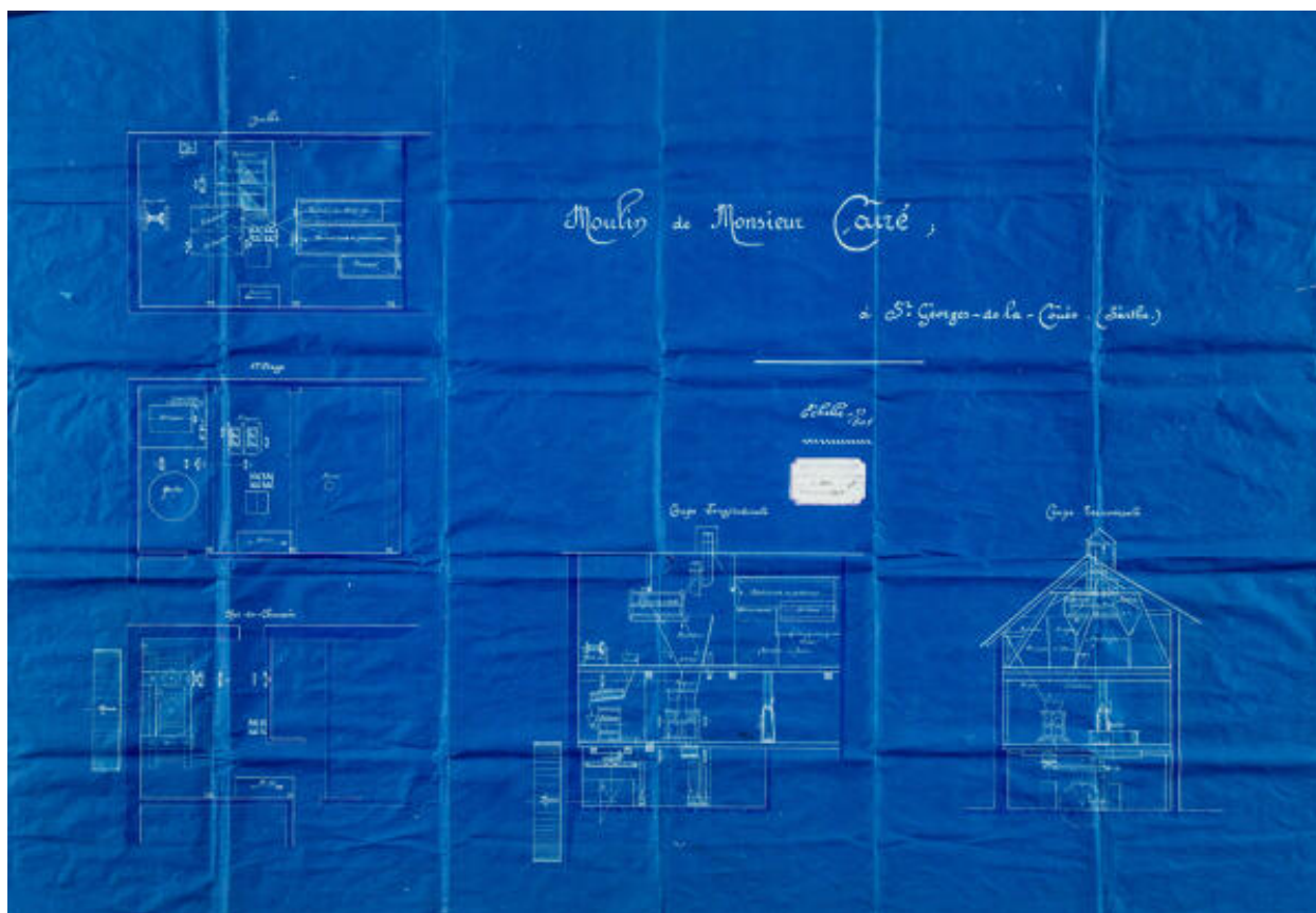
Projet de modernisation avec installation de nouvelles machines : plan et coupes, 1907.
