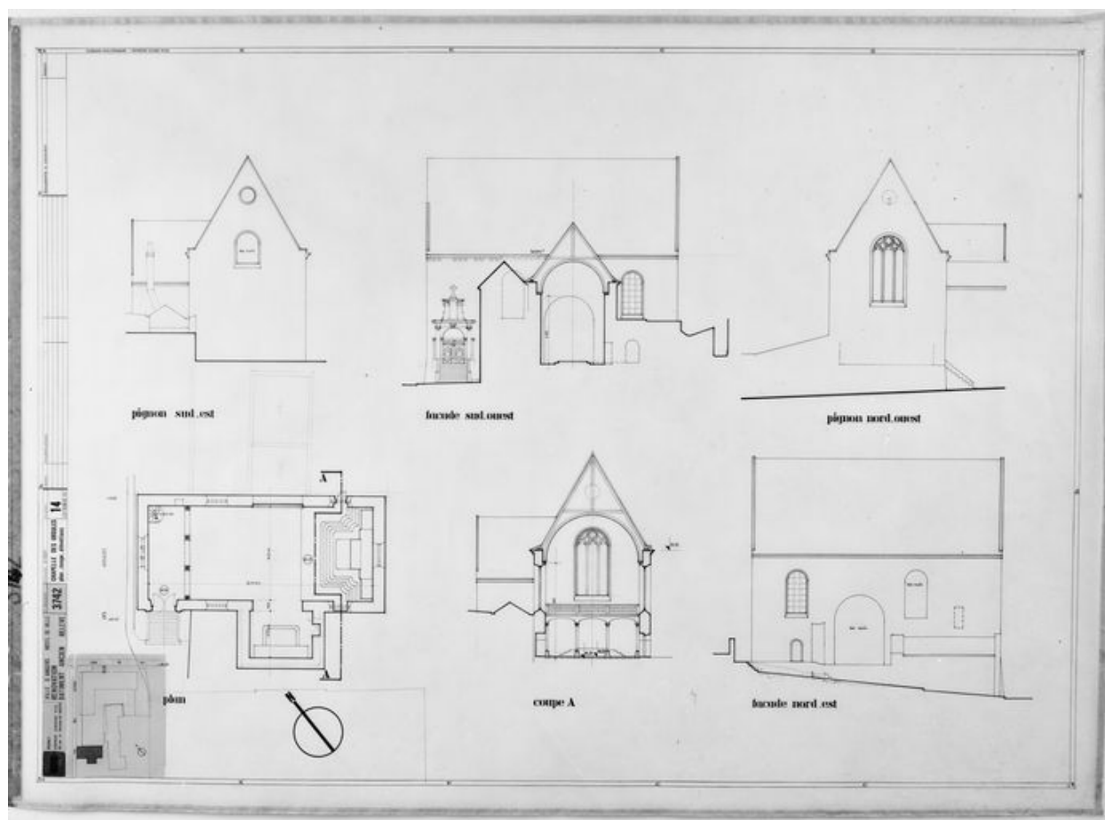
Eglise : plan, élévations, coupes transversale et longitudinale, dessin par P. Mornet, 1974.
