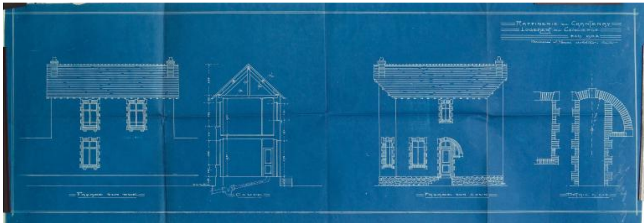
Raffinerie de Chantenay. Logement de concierge. Élévations, coupe et détail de la porte. 1921.
