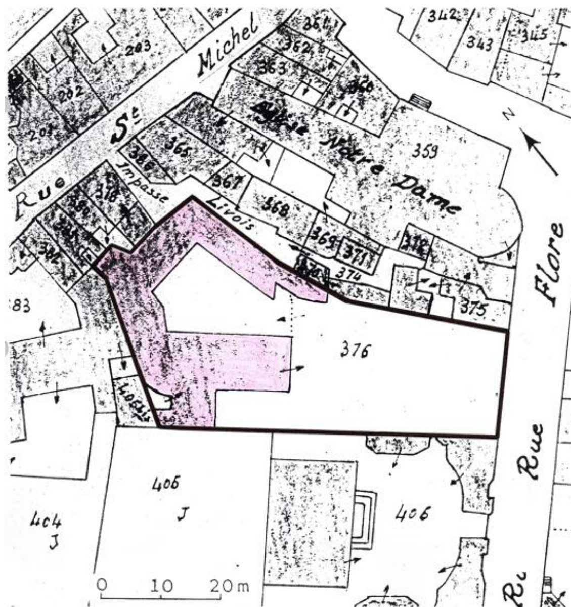
Plan-masse et de situation. D'après le plan cadastral, 1840, section H1, parcelle 376, éch. 1 : 1 000. Augmenté.
