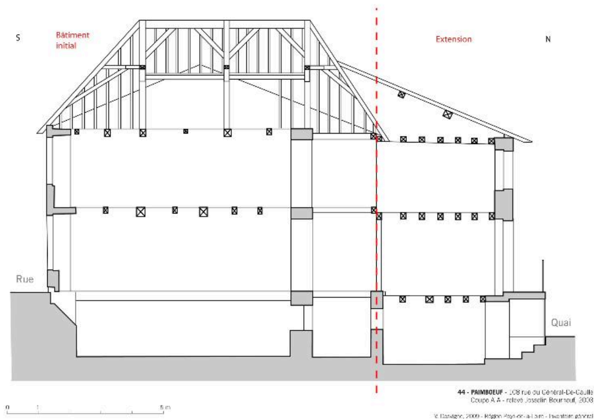
Maison, 108 rue du Général-de-Gaulle : coupe nord-sud.
