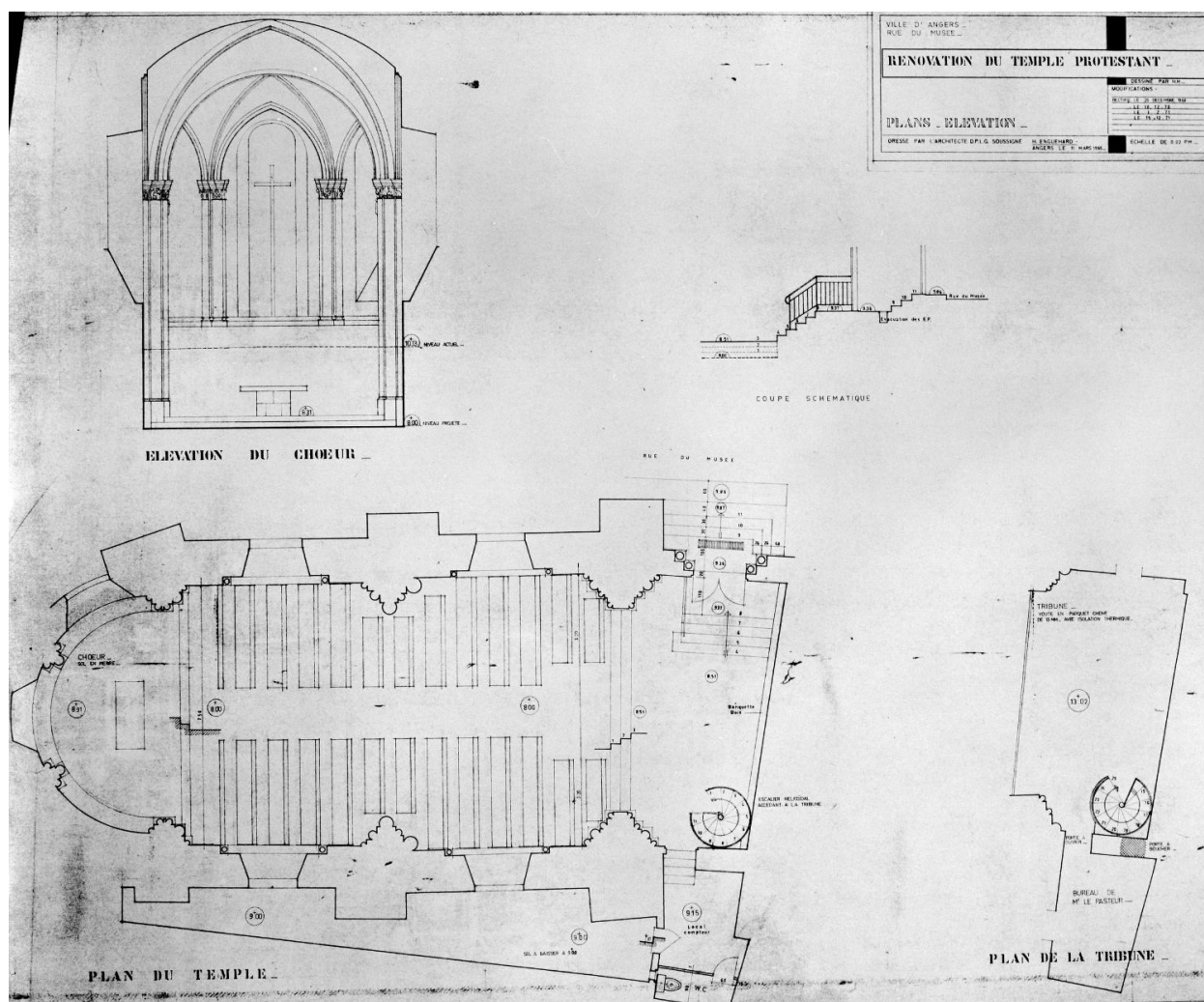
Plan du temple (église Saint-Eloi), plan de la tribune et élévation intérieure du choeur, par H. Enguehard, 1966.
