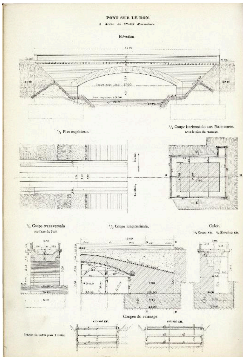
Plan, élévation et coupes du pont sur le Don, 1877.
