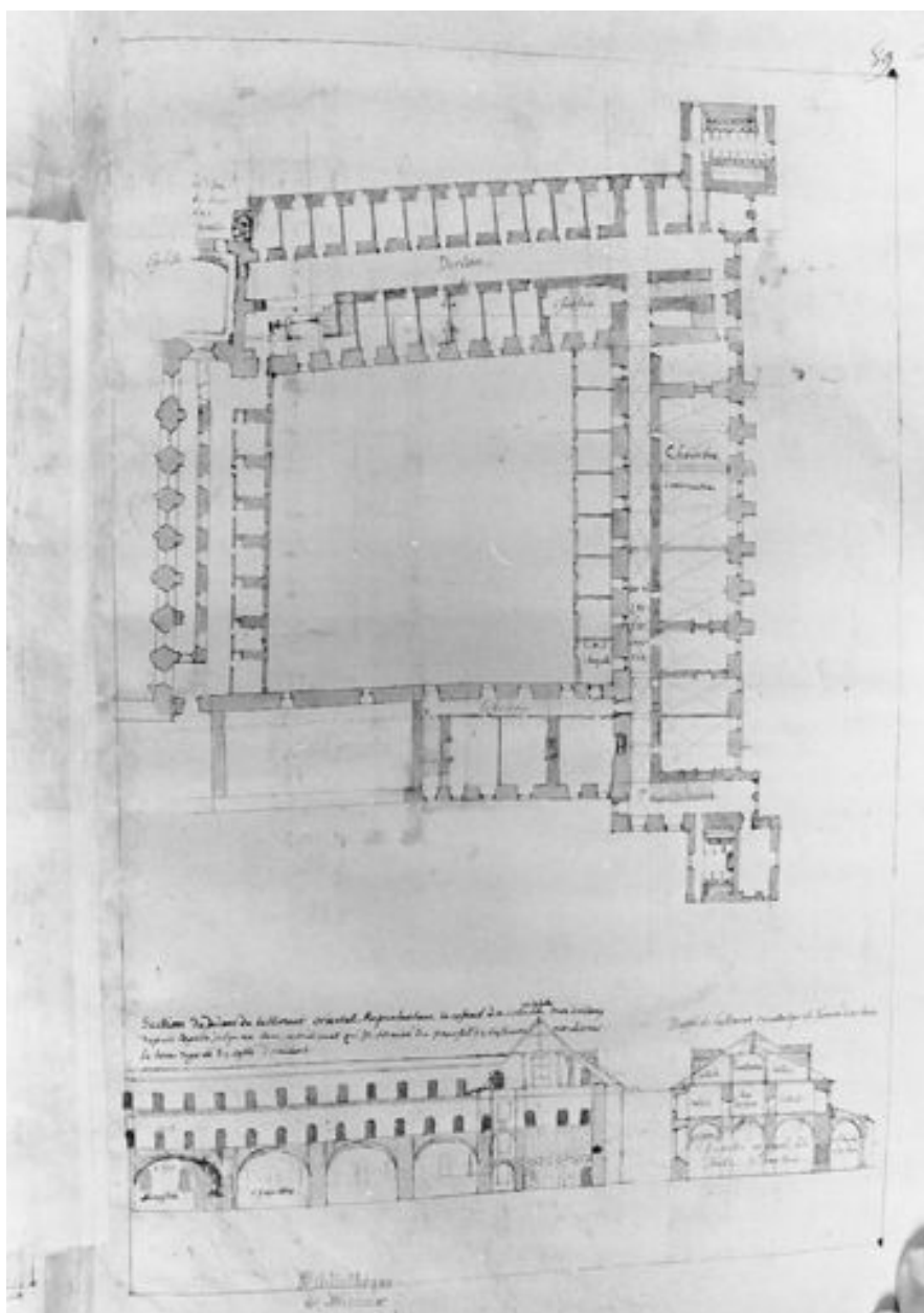
Projet global de reconstruction, attribué à Marc Rivard : plan d'étage (au-dessus du réfectoire) et coupe longitudinale et transversale de l'aile orientale des dortoirs, 1680. (Bibliothèque municipale de Meaux ; Ms. 44, f. 89 bis r°).
