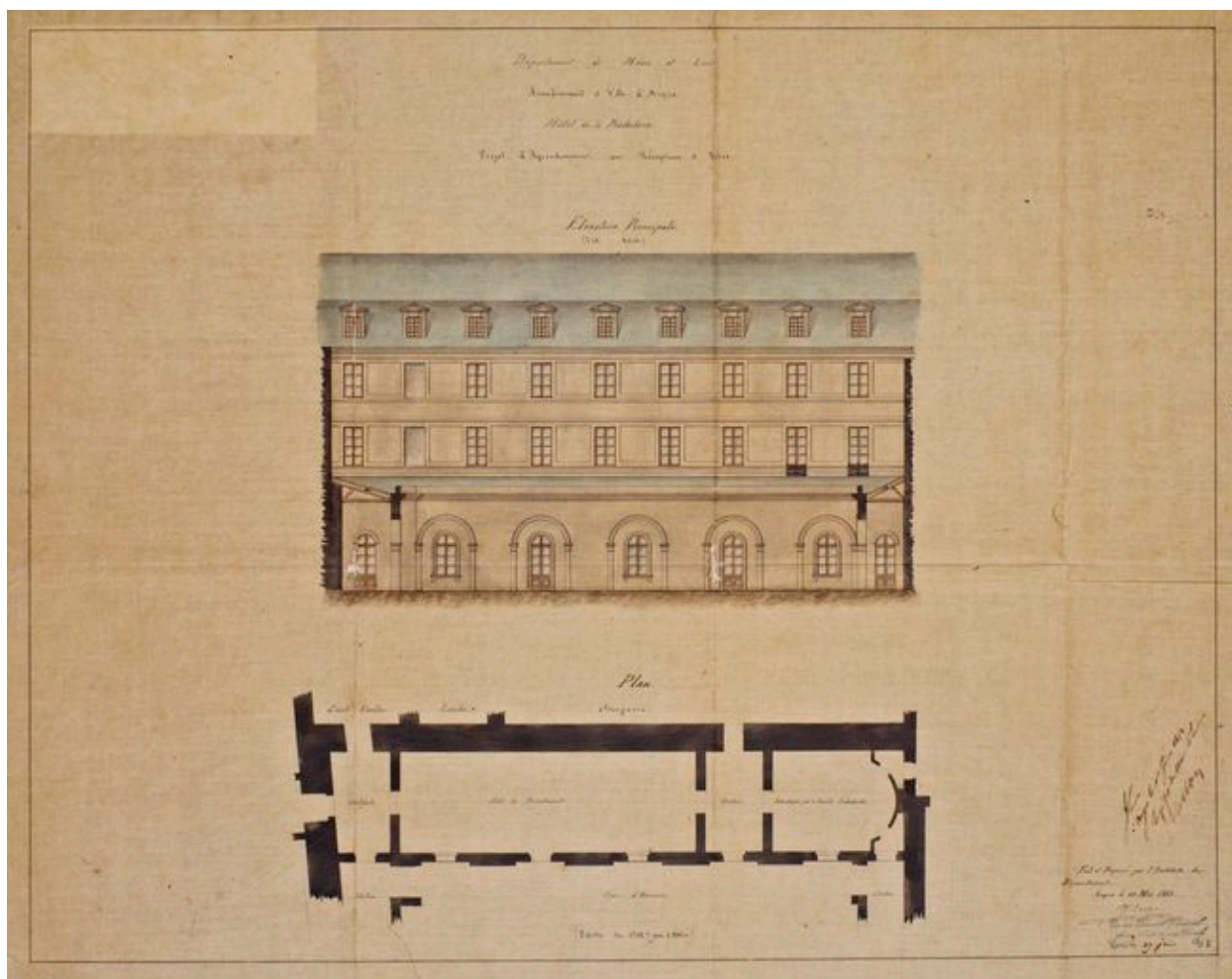
Projet d'agrandissement pour réceptions et fêtes. Élévation (état actuel). Plan [au rez-de-chaussée], 1853. Dessin à la plume et aquarelle, éch. 1 : 200e. (Archives départementales de Maine-et-Loire ; N 1769).
