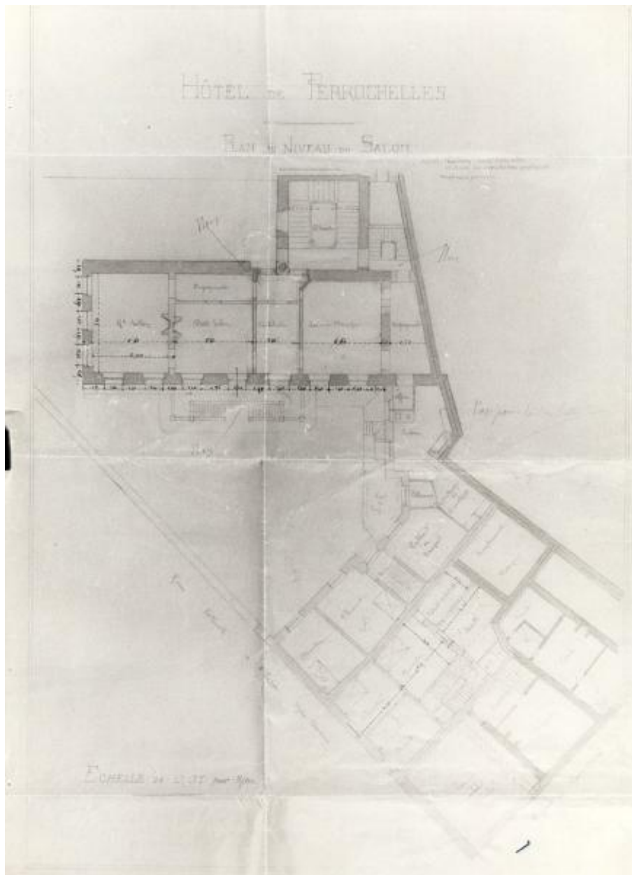
Plan du rez-de-chaussée, projet de remaniement et d'extension (en bas à droite), par l'architecte Auguste Martin. Dessin, fin 19e siècle, éch. 1:100e. (Collection particulière, Pousset).
