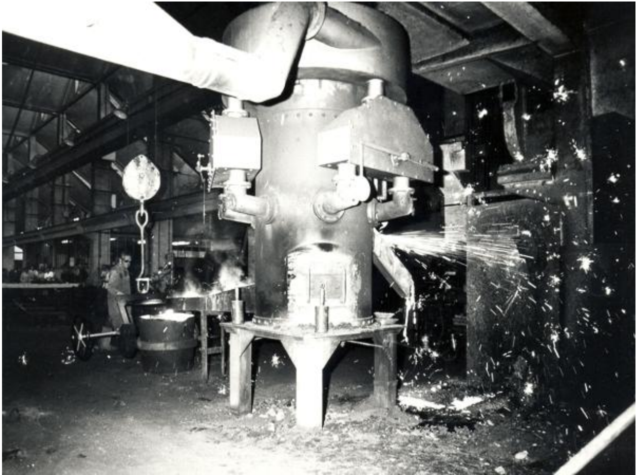
Atelier de fonderie : base du cubilot gauche. Tuyère de coulée du laitier à droite.
