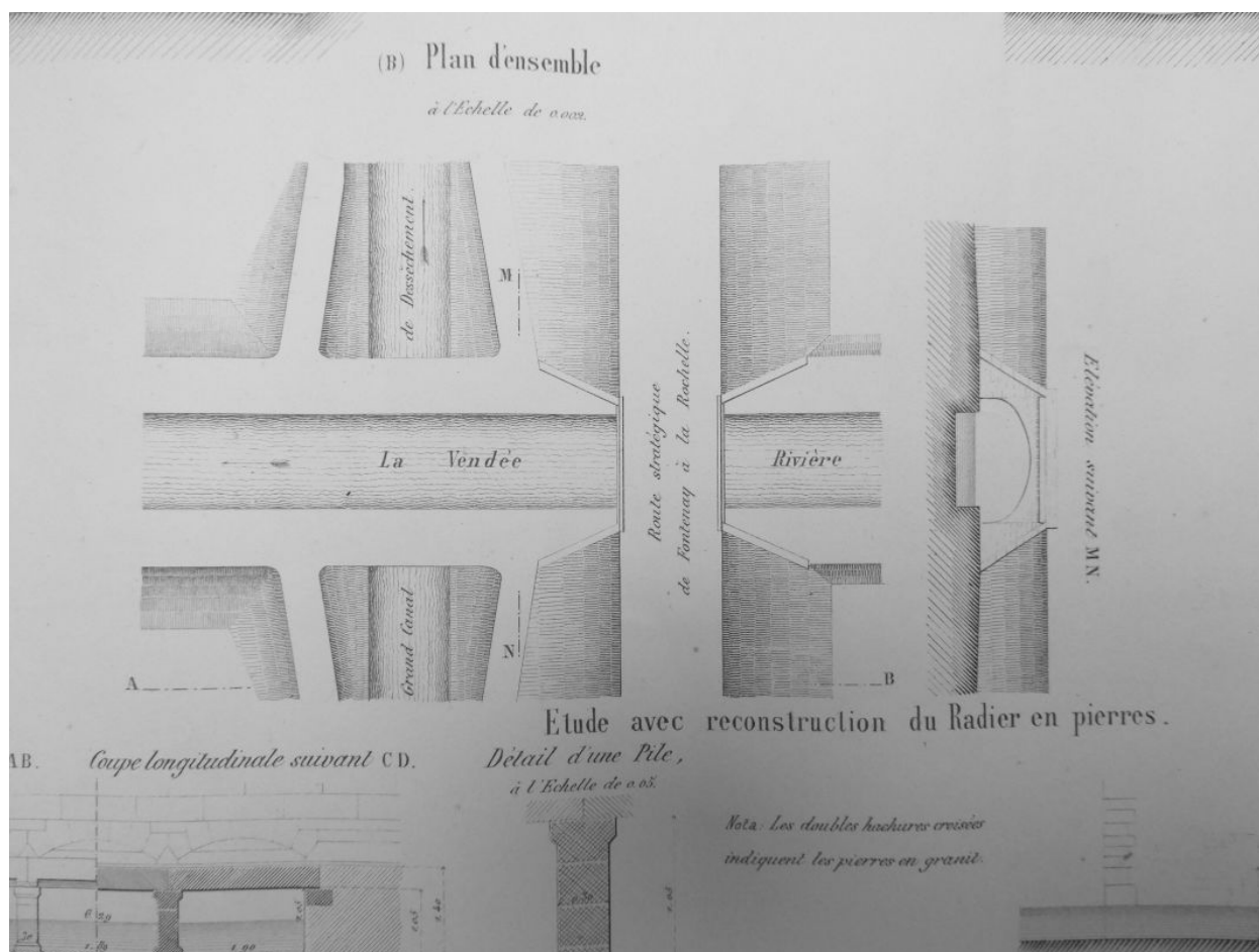
Plan du Gouffre vers 1894 : plan et élévation sud.
