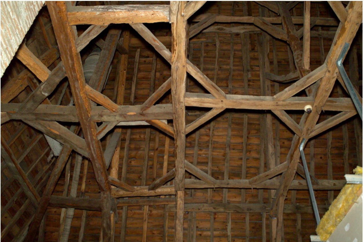
Charpente de l'aile est.
