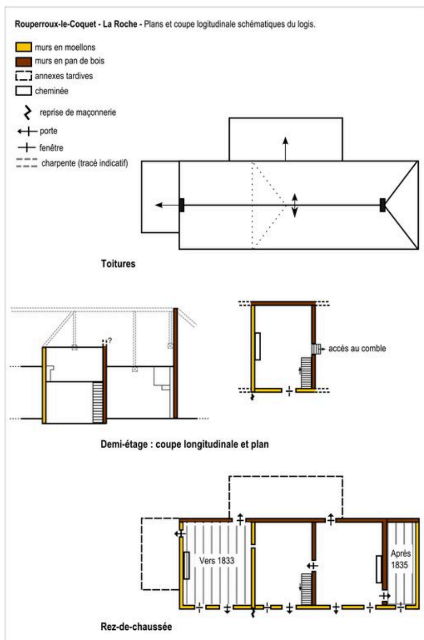
Plans et coupe longitudinale schématiques du logis
