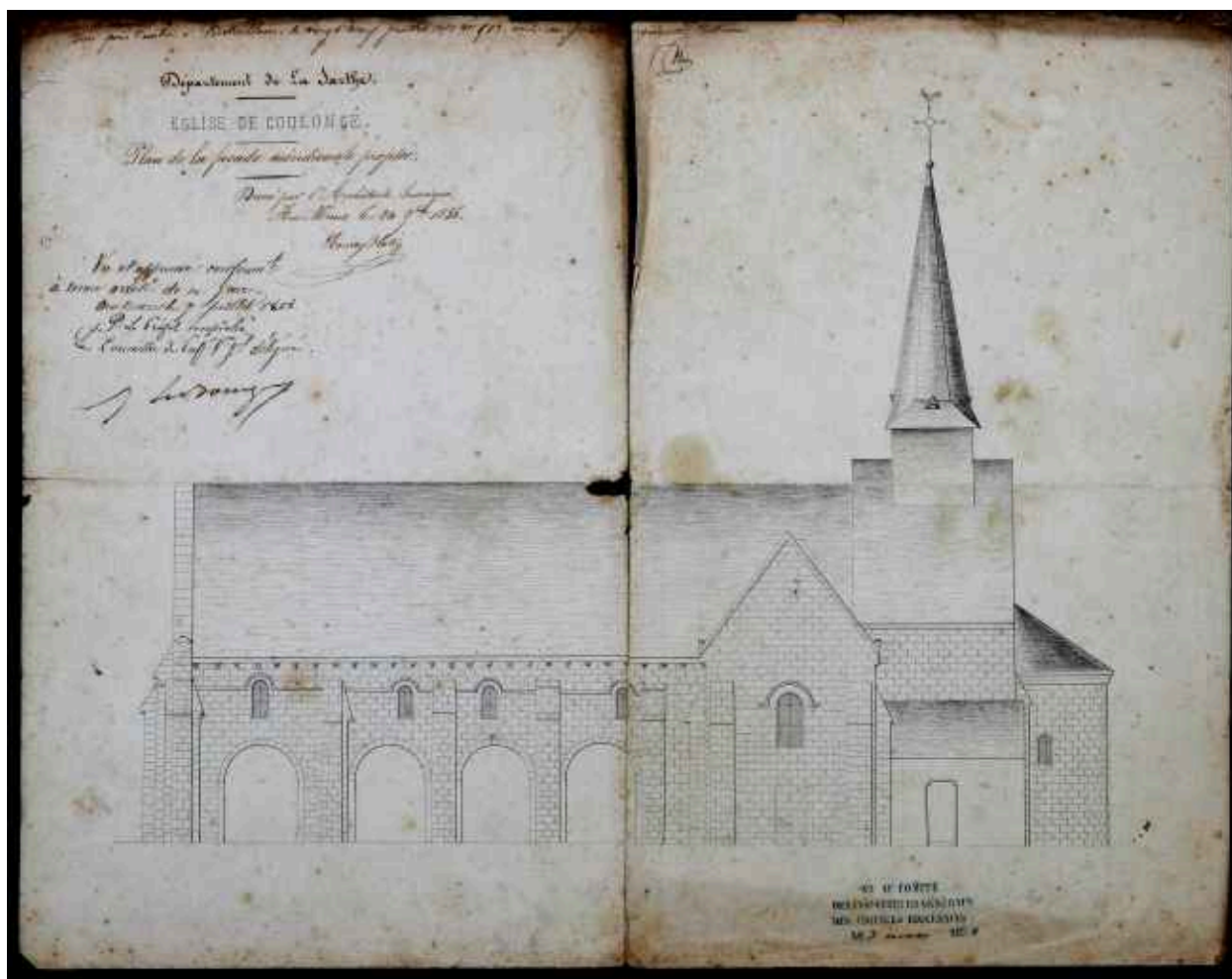
Élévation de la façade méridionale projetée, 1858.
