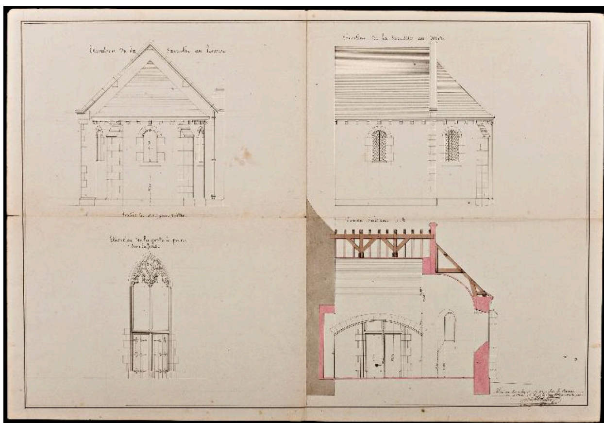
Elévations et coupe du projet de sacristie néo-romane non réalisé. 1864.
