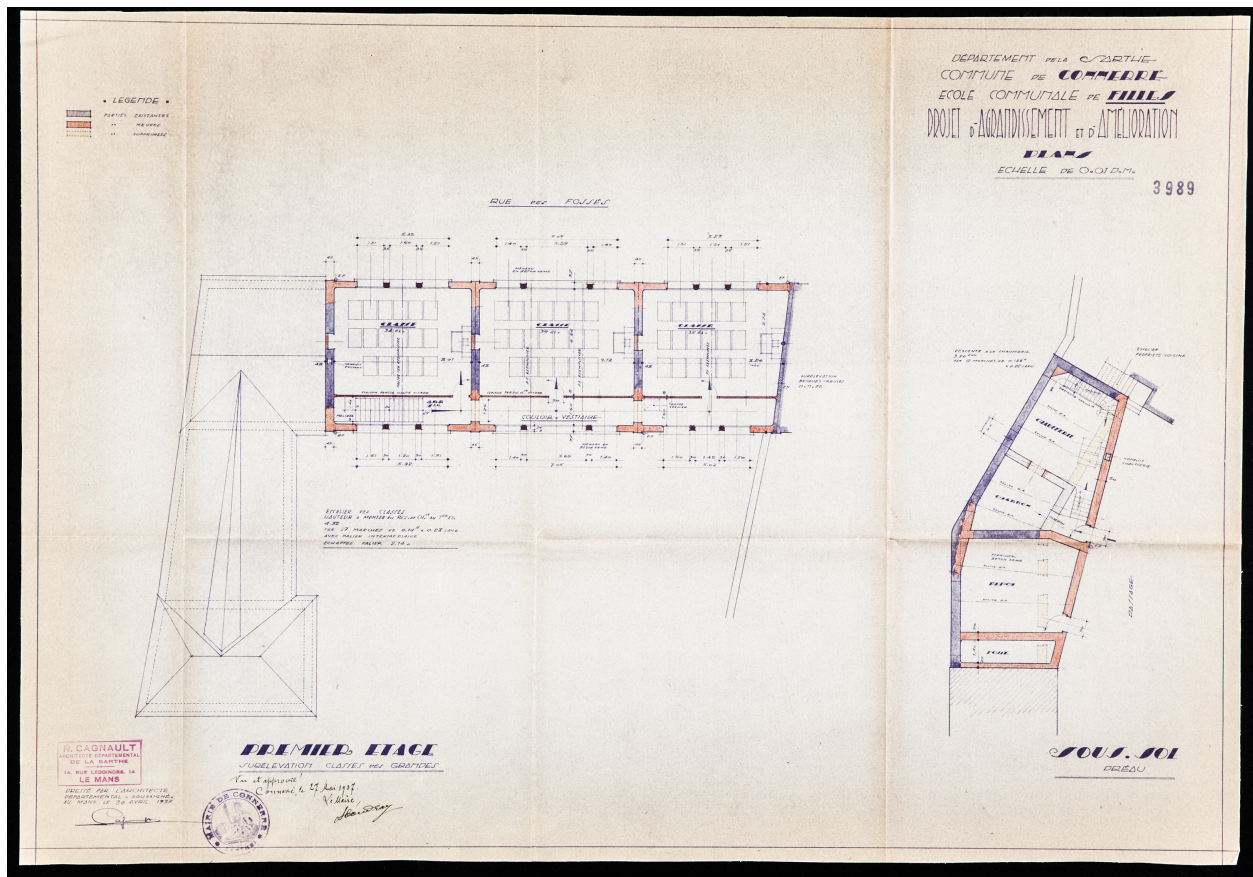
Le projet d'agrandissement de l'école de filles (non réalisé), par R. Cagnault, 1937, plans du premier étage.
