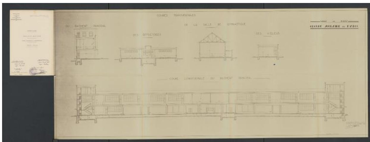
Coupe de l'école primaire Jules-Ferry, 1938.
