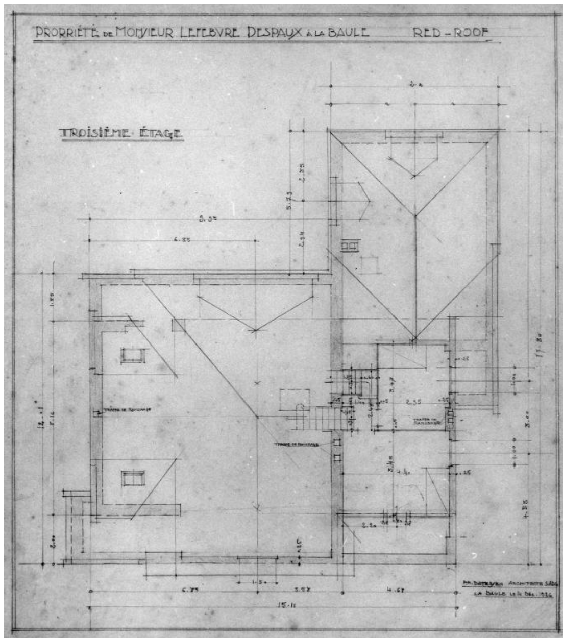
Plan du 3e étage au 1/50e de la villa Red-Roof pour M. Lefebvre Despeaux en 1926.
