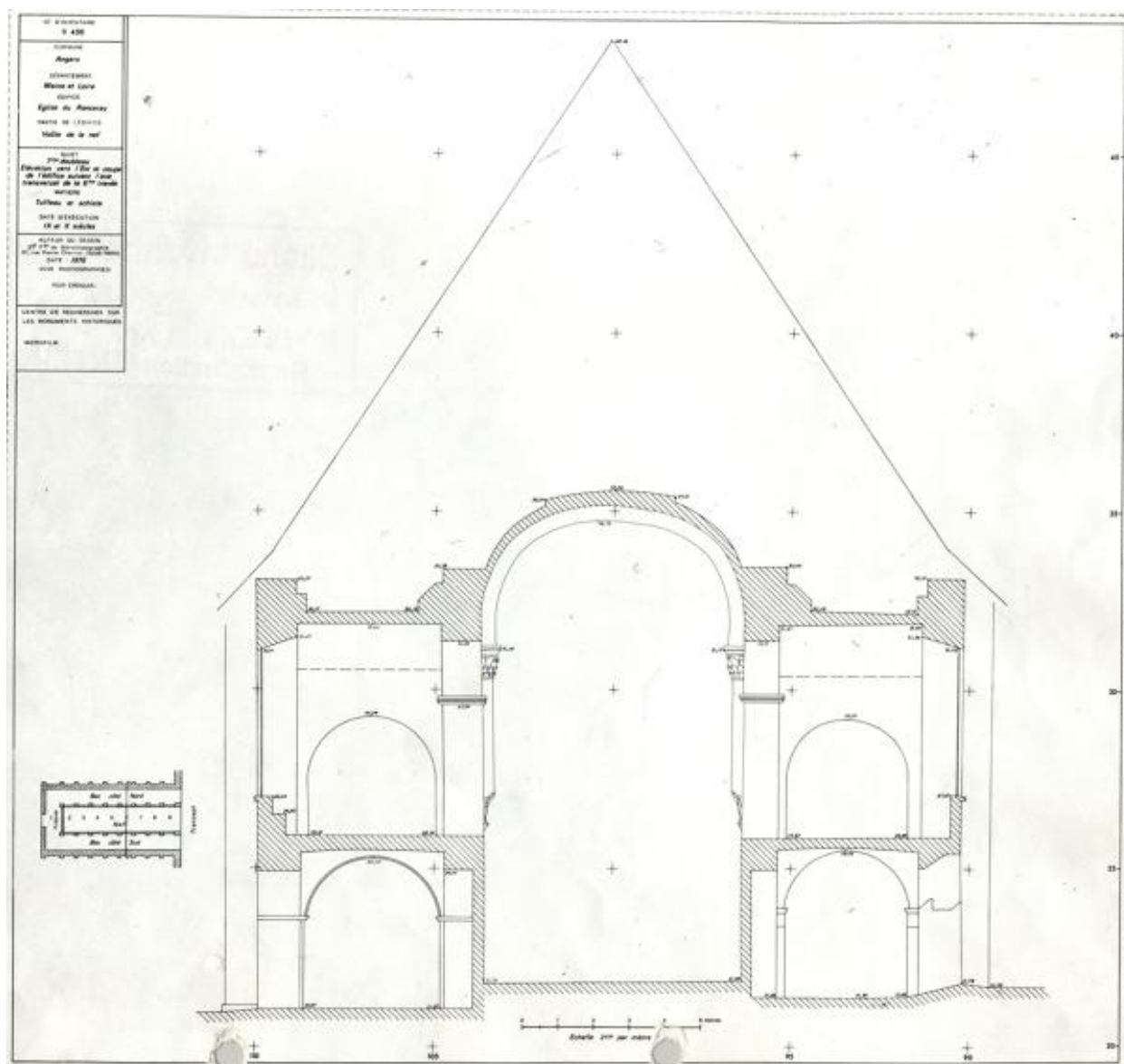
Eglise, coupe transversale, relevé stéréotopographique, [v. 1976].
