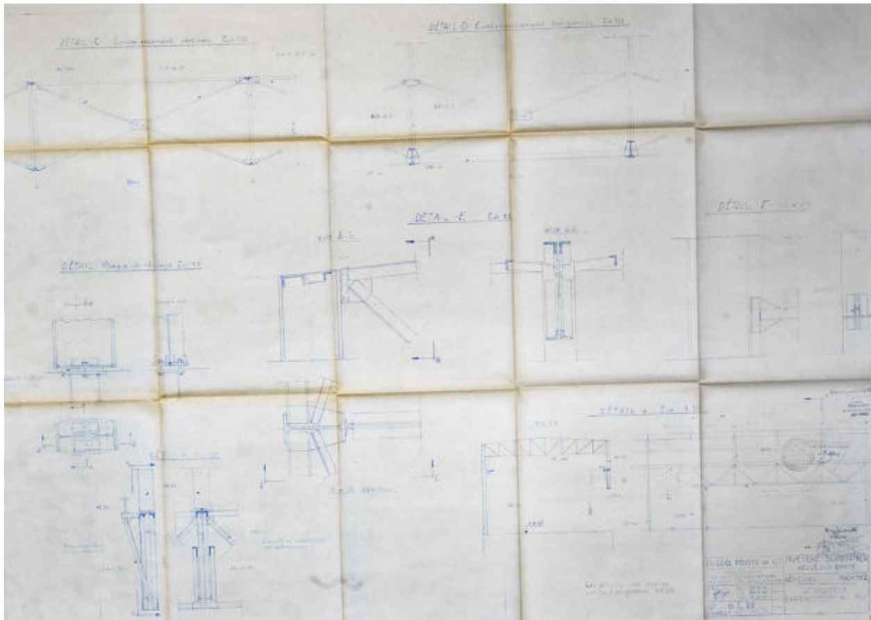
Détail de la charpente du bâtiment de la machine à papier (groupe 2) édifié en 1964.
