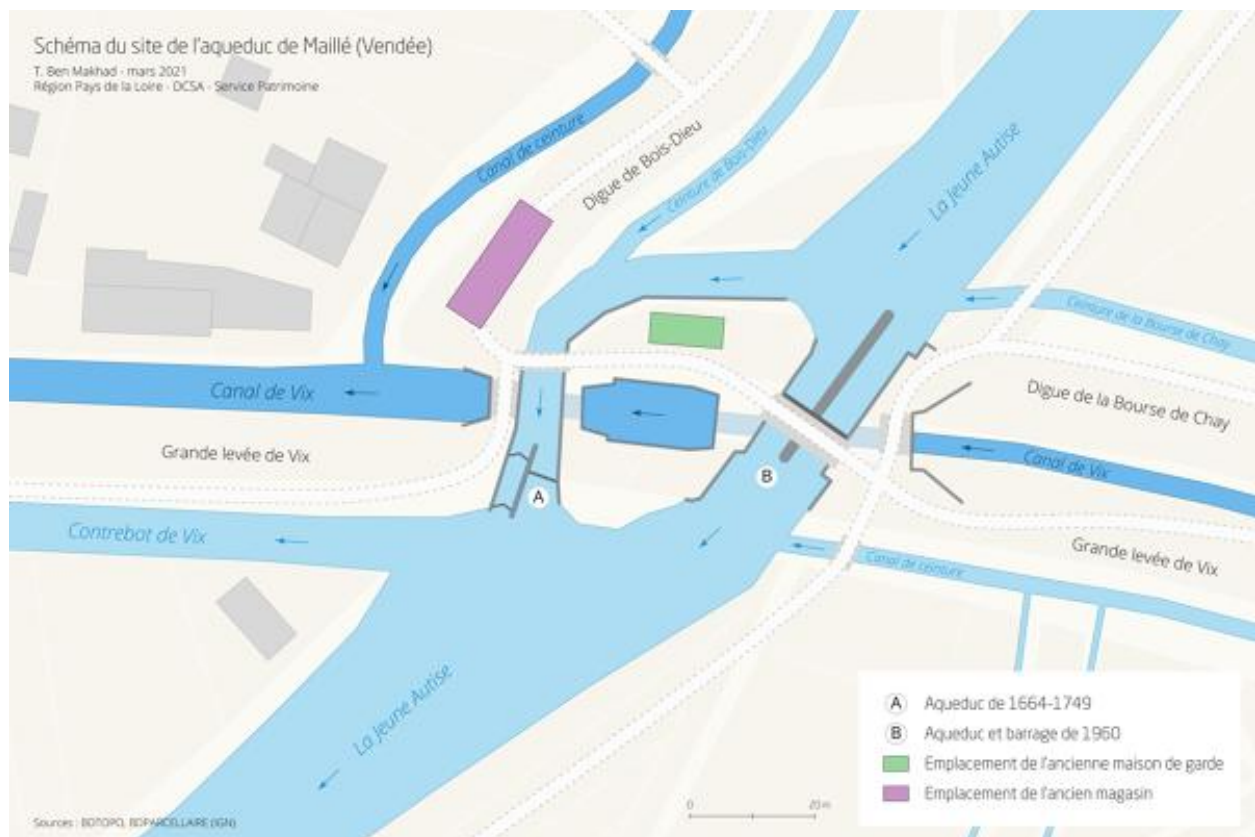
Schéma du site de l'aqueduc de Maillé (Vendée)
