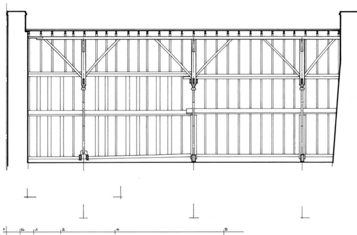
Coupe longitudinale de la charpente. Relevé R. Bodier, 2010.
