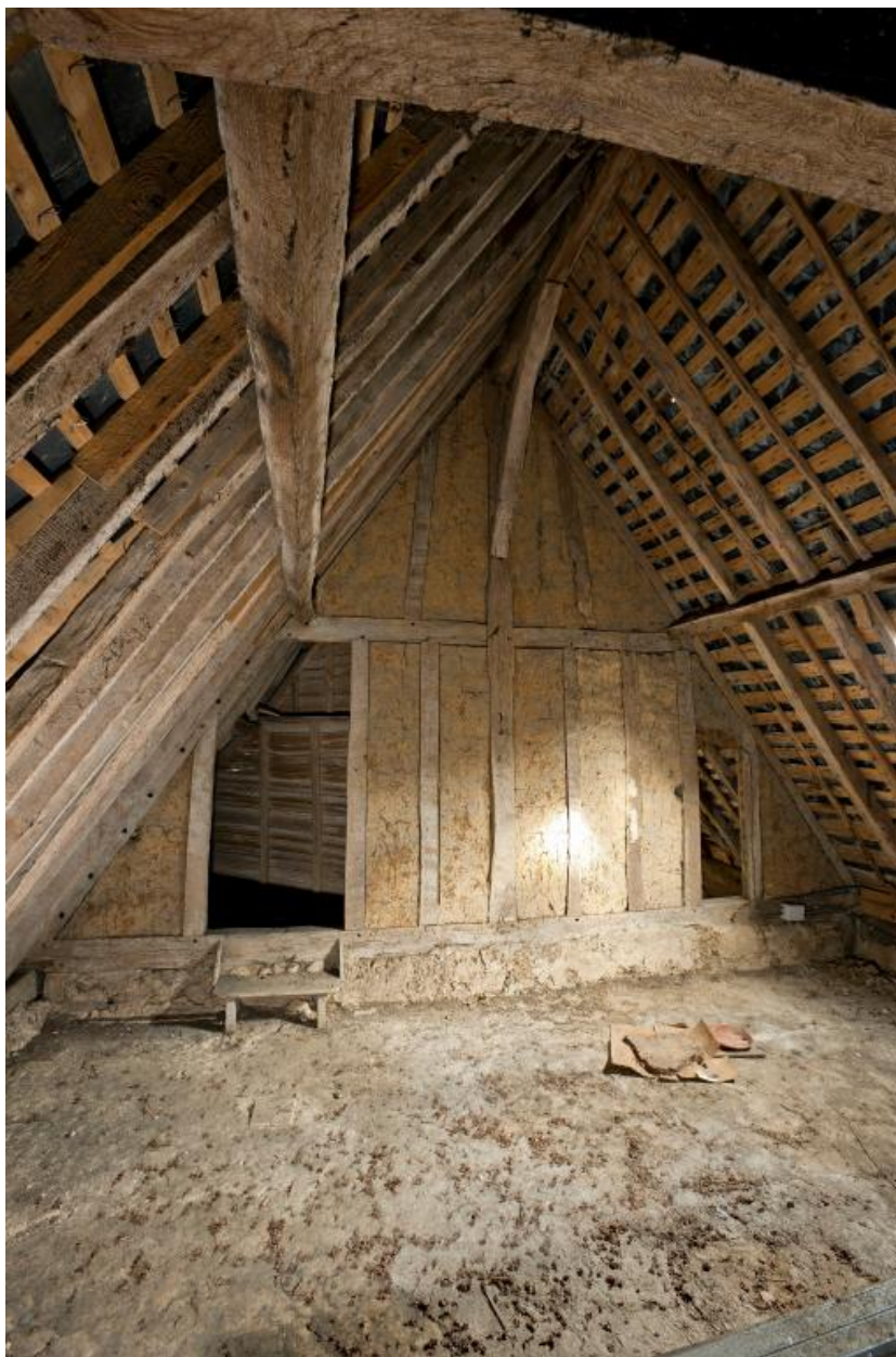
Comble avec cloison centrale.
