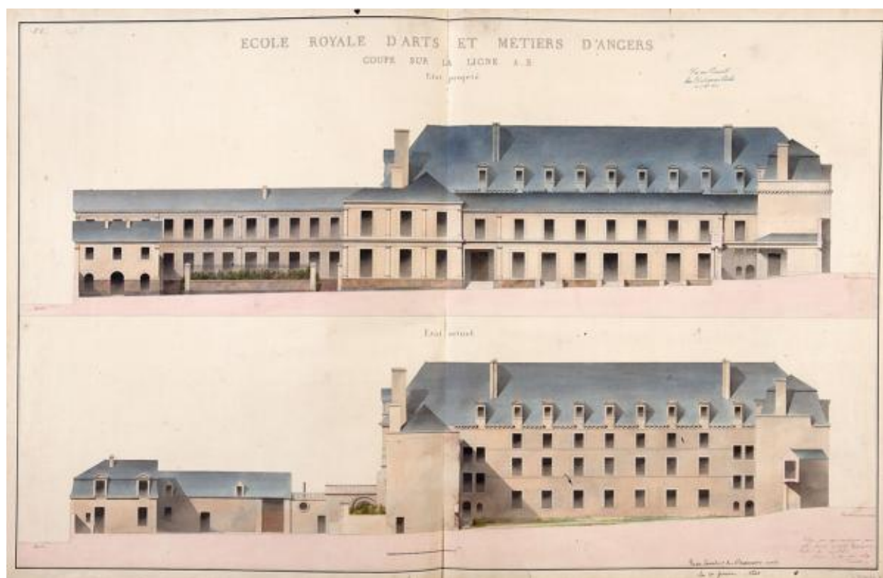
Ecole royale des Arts-et-Métiers d'Angers. Coupe sur la ligne AB [élévation d'ouest en est, le long de la face nord de l'aile nord du cloître]. Etat actuel. Etat projeté, par Ch.-E. Isabelle, 1839. Ensemble de la planche.
