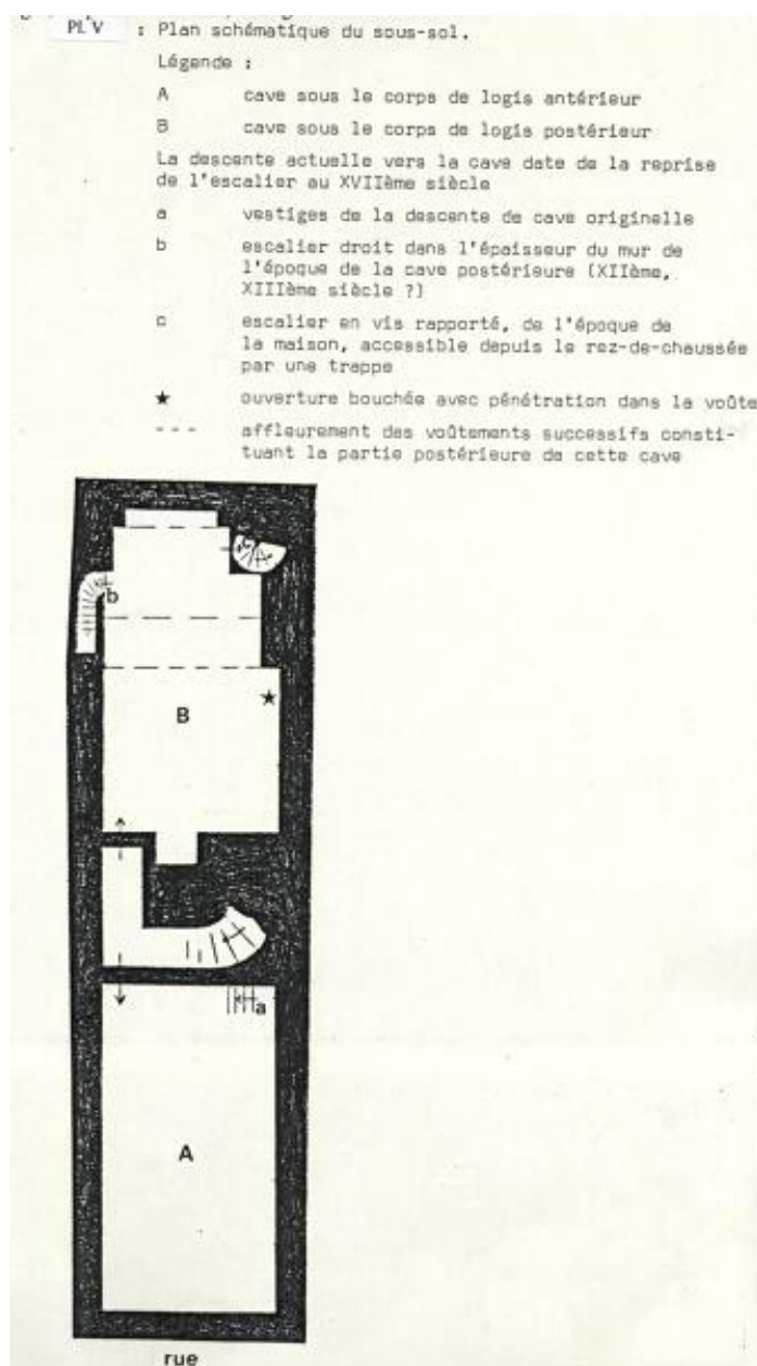
Plan schématique du sous-sol.
