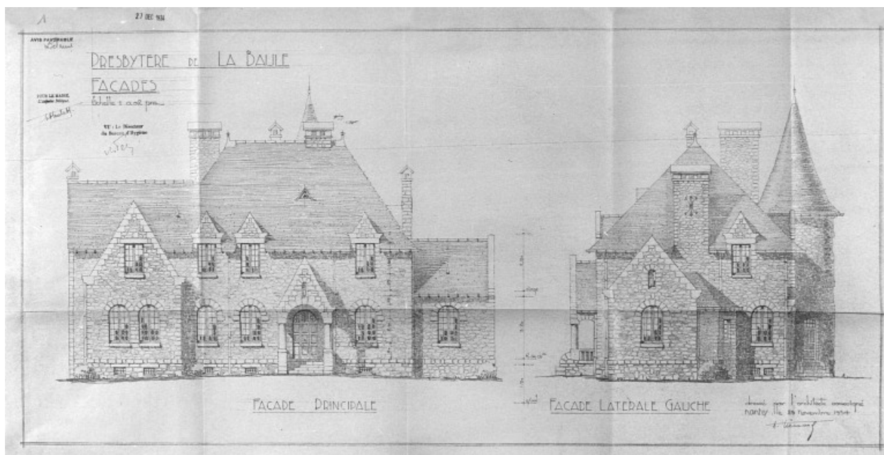
Presbytère de La Baule : façades nord et ouest au 1/50e.
