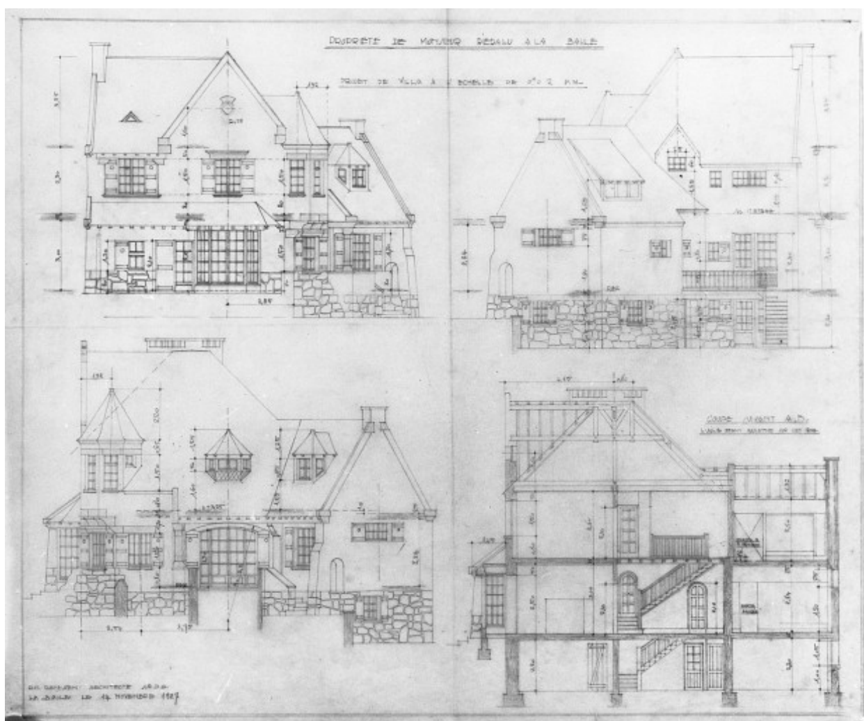
Façades et coupe au 1/50e de la villa Saint-Corentin pour M. Piedalu en 1927
