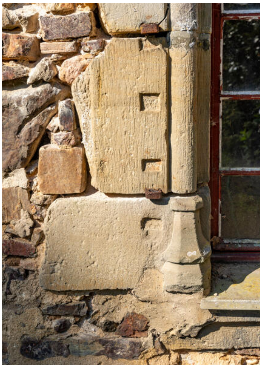
La grande fenêtre du rez-de-chaussée, détail de l'encadrement.
