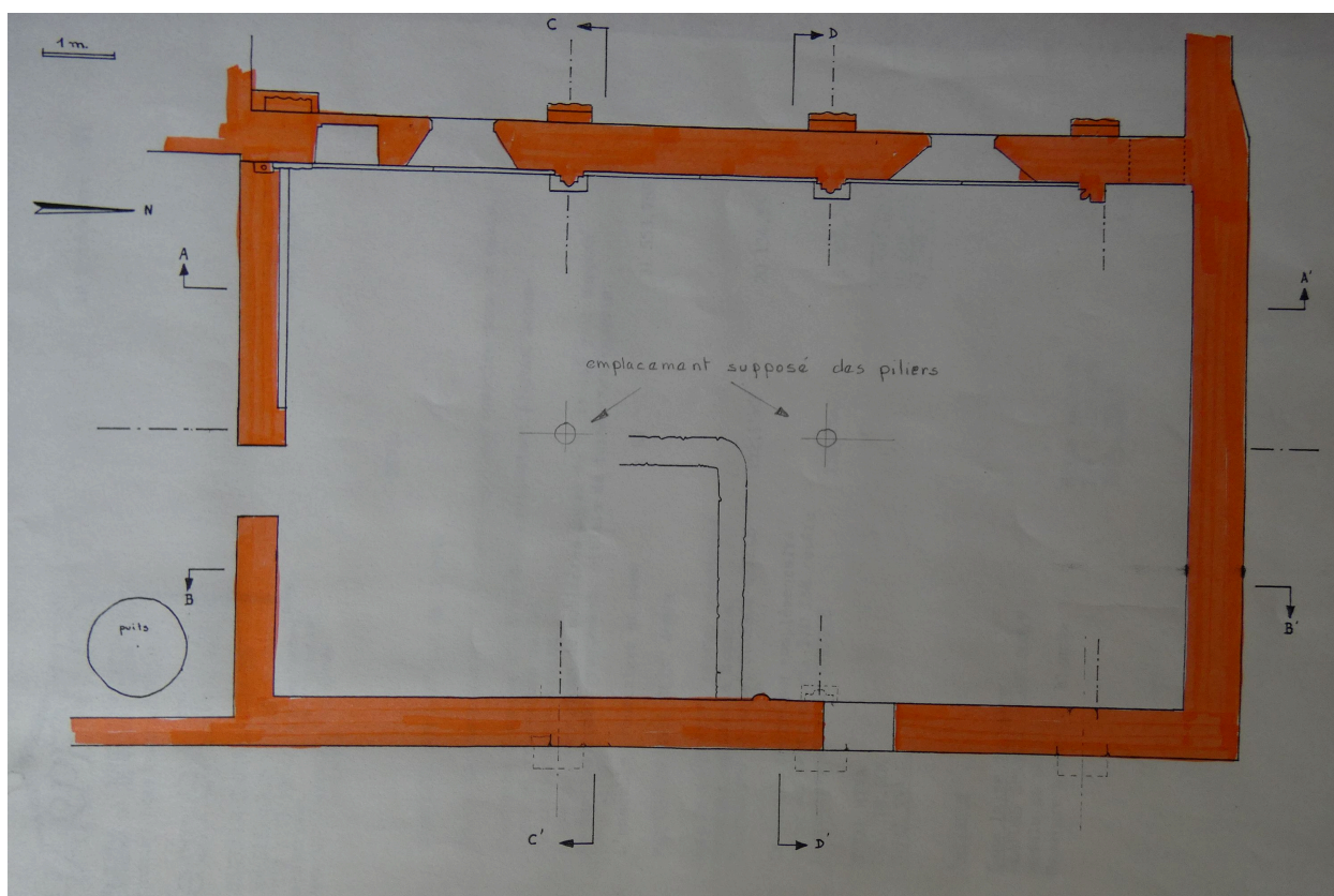
Plan des vestiges de la chapelle de Lesson, s. d. (fin du 20e siècle).
