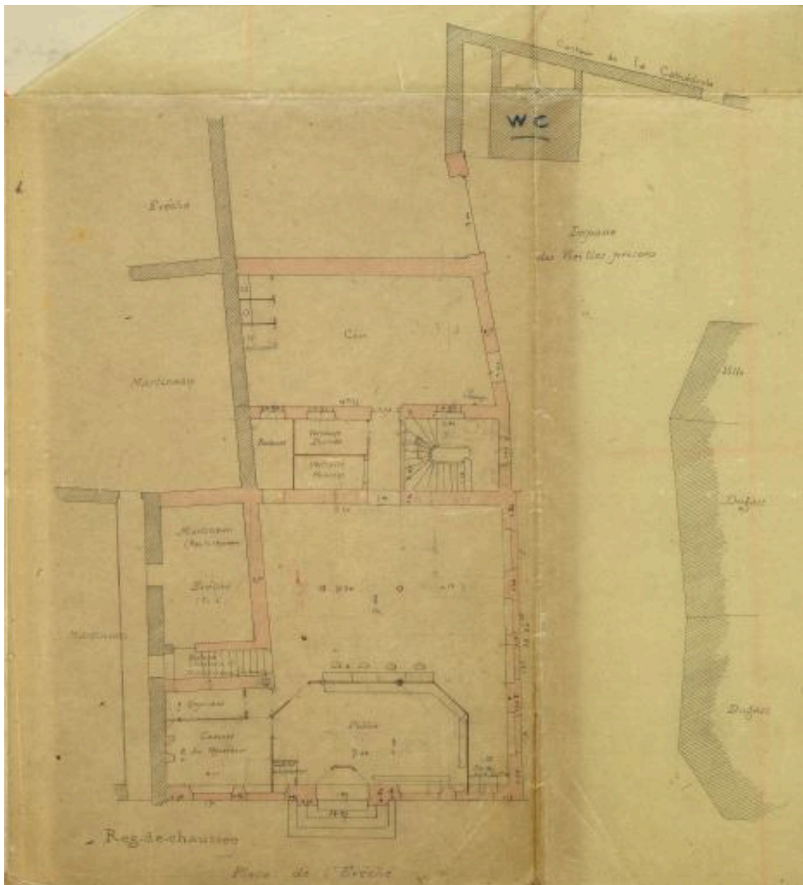
Plan du rez-de-chaussée par Bordelais, en 1898.
